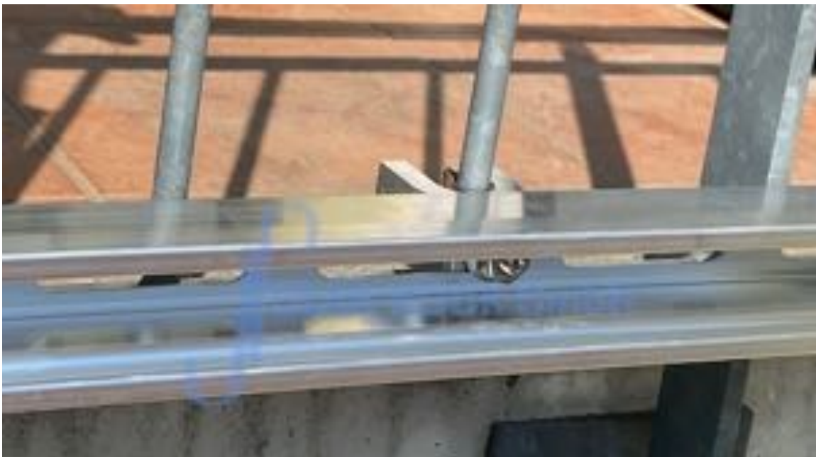
Abb.g 13/Montageschiene und Spezialklemme von außen
