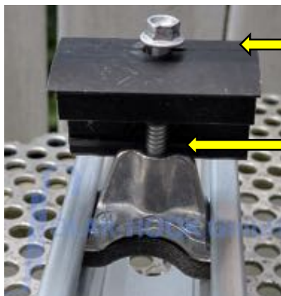
Abb. 16/ vormontierte Modul-Endklemme
