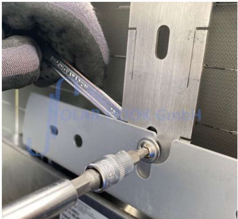
Abb. 7/Wechselrichter am SOLAR-HOOK Befestigungsbügel anschrauben
